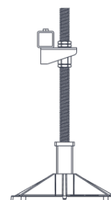
Komplettes Bein mit verlängerter Gewindestange Höhenverstellung: 335 - 660 mm
