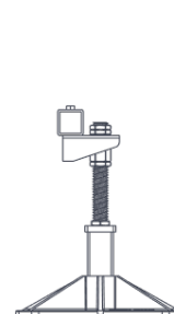
Komplettes Bein Höhenverstellung: 335 - 440 mm
