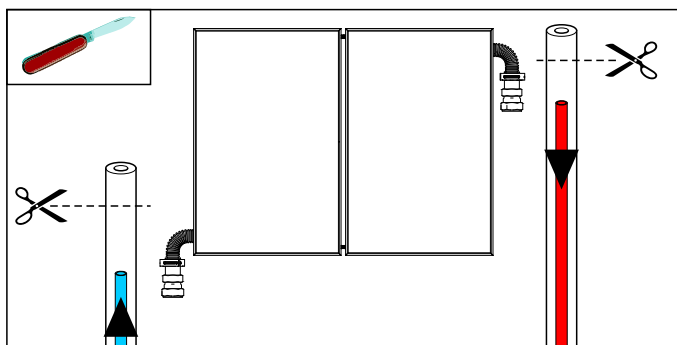
Bild 4-17 Arbeitsschritt 5
