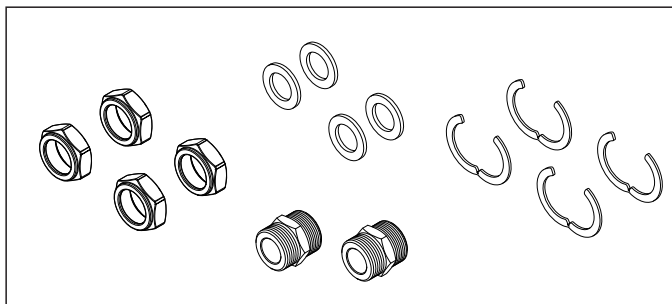
Bild 3-7 CON XP16 / CON XP20 (optional)
