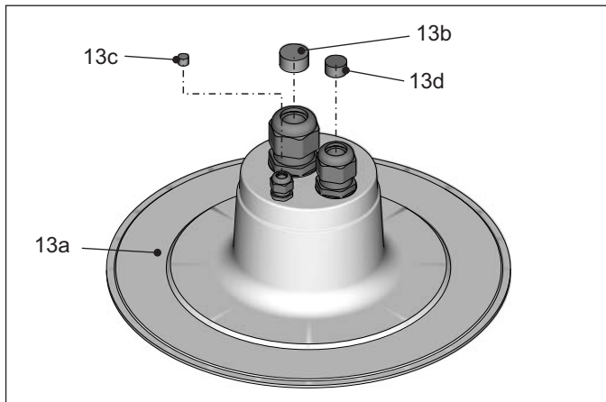
13a Flachdachdurchführung CON F
