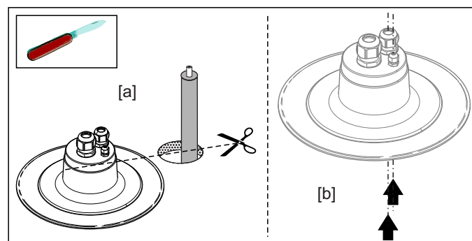
Bild 4-4 Arbeitsschritte 5a und 5b
