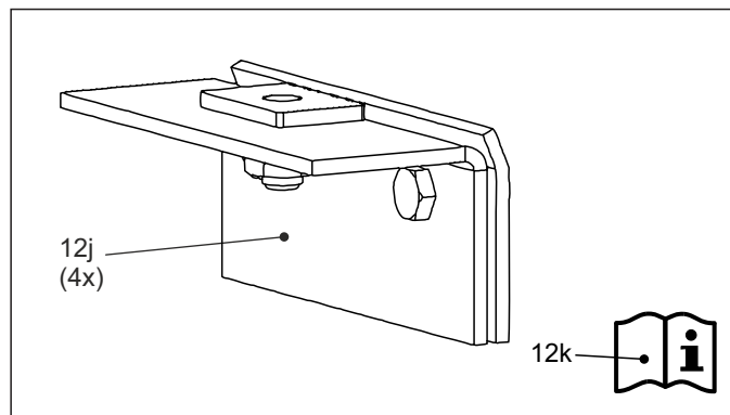
Bild 3-14 FIX BD
