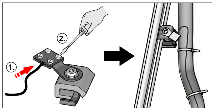
Bild 4-20 Arbeitsschritte 1+2
