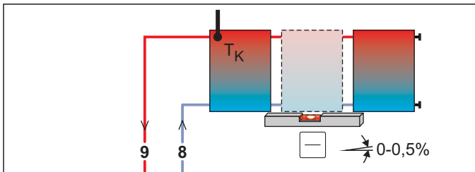
Bild 4-2 Gleichseitig angeschlossenes Solar-Kollektorfeld (max. 3 Solar-Kollektoren)
