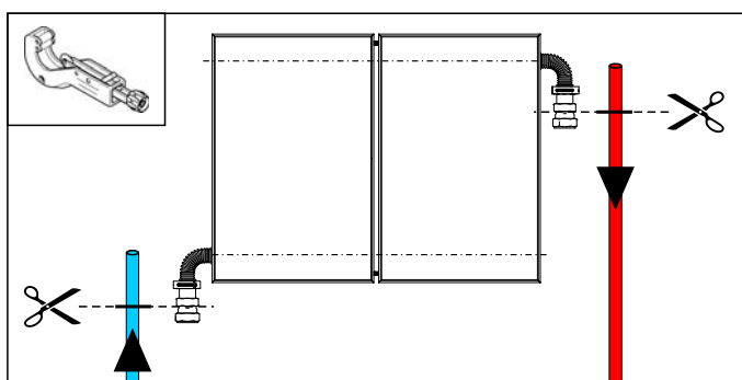
Bild 4-16 Arbeitsschritt 4
