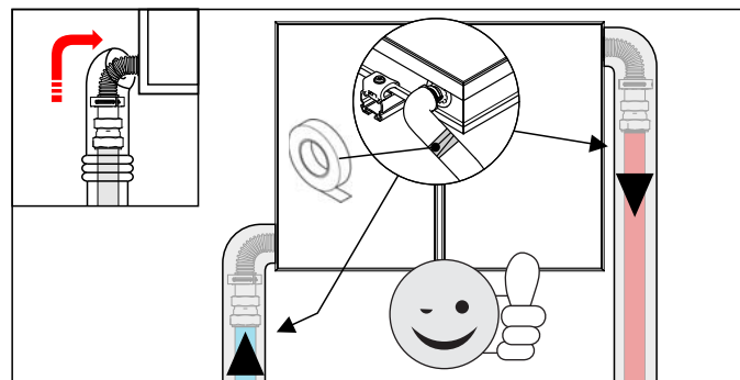
Bild 4-19 Arbeitsschritt 7
