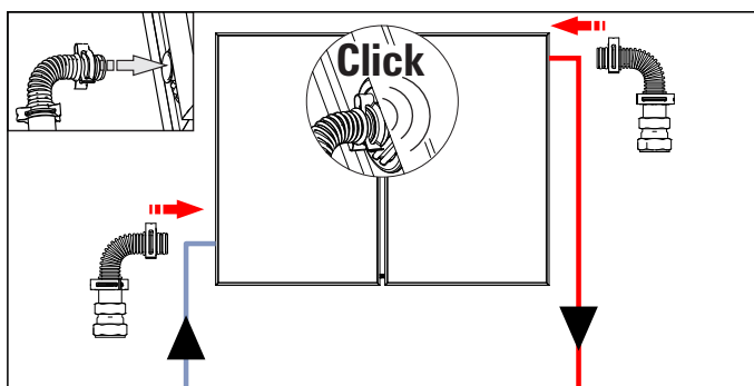
Bild 4-14 Arbeitsschritt 2
