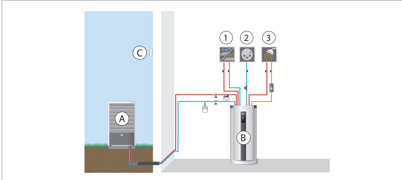
Abb. 42: Beispiel Hydraulikschema
