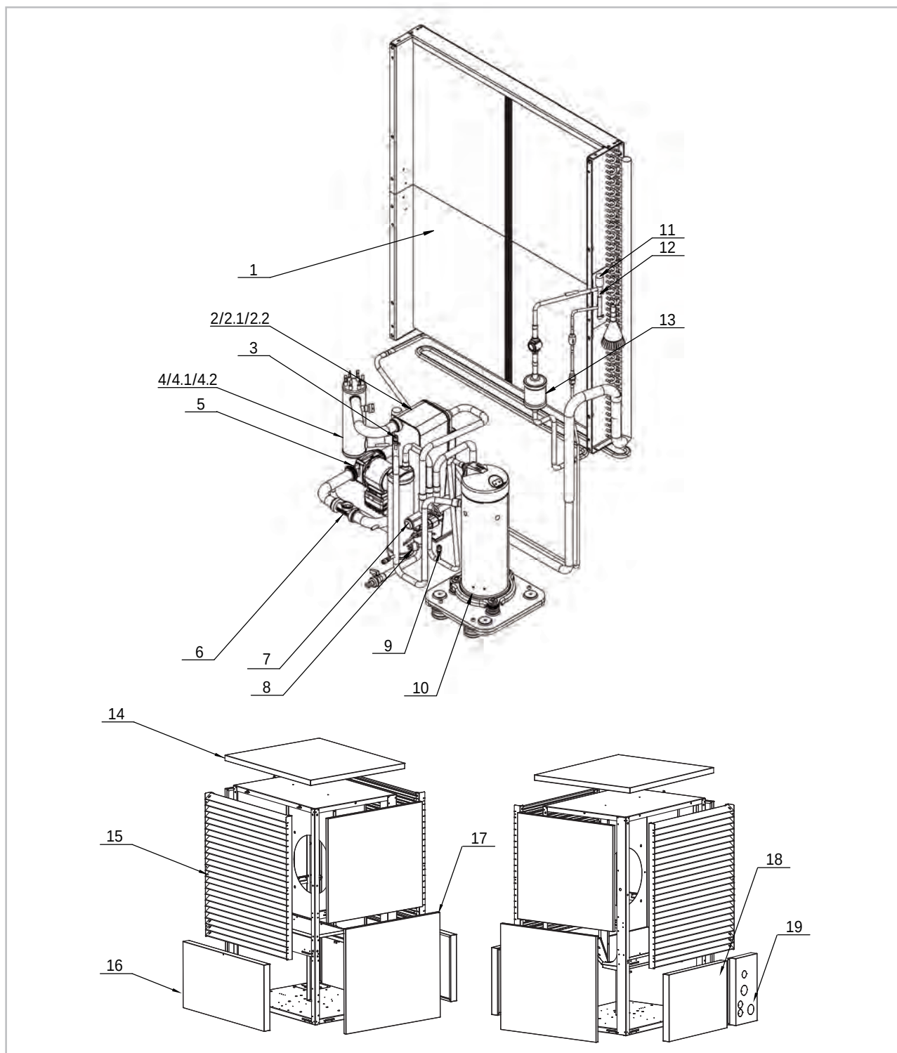
Abb. 46: Explosionszeichnung
