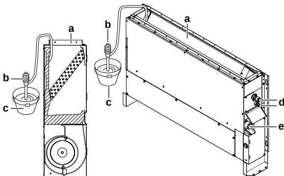
a Luftauslass b Tragbare Pumpe c Behälter d Kältemittelleitungen e Entleerungsauslass
