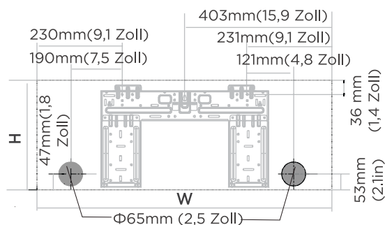
Abmessungen des Innengeräts (BxH): 805mm(31,7 Zoll)x295mm(11,6 Zoll)
