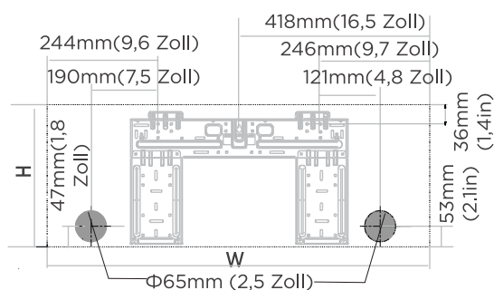
Abmessungen des Innengeräts (BxH): 835mm(32,9 Zoll)x295mm(11,6 Zoll)
