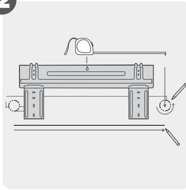
Bringen Sie die Montageplatte an
